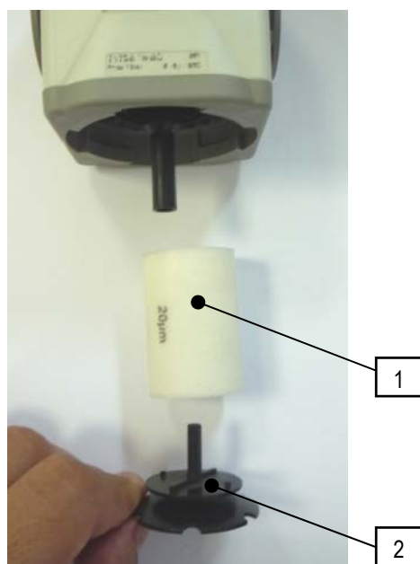
Детали фильтра: 1 – сменный фильтр-элемент, 2 – стопорный винт
