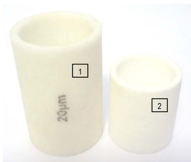
Примеры фильтр-элементов: 1– RS/1703/262 (высота 45 мм), 2– RS/1703/13 (высота 35 мм).
